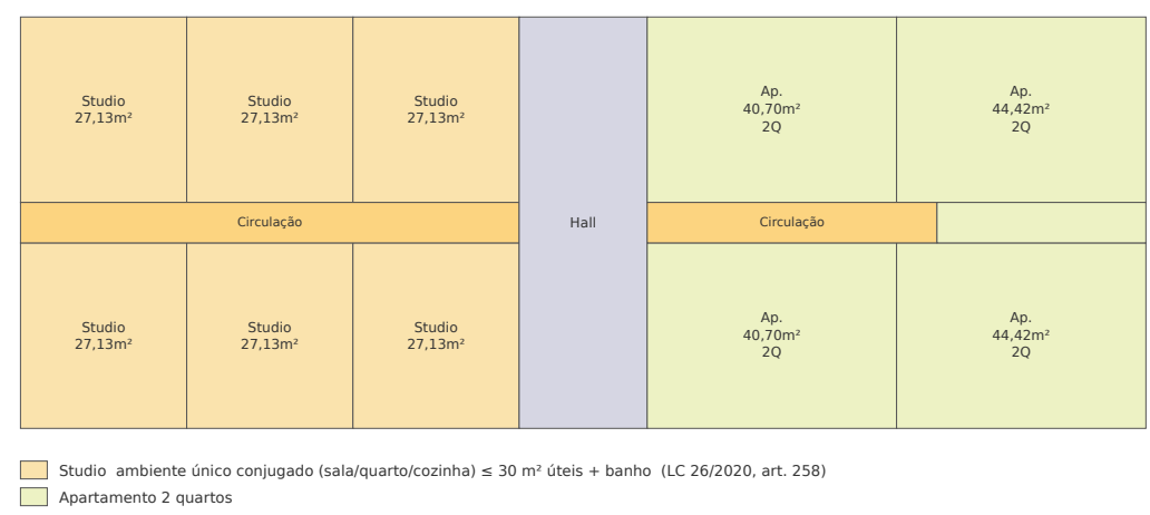
Pavimento Tipo misto (cada torre)
